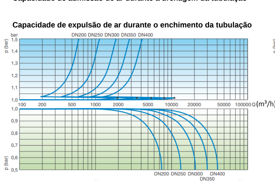
Capacidade de admissão de ar durante a drenagem da tubulação
